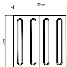
Sinalização Tátil Direcional - Modulação do Piso SEM ESCALA (Fonte: ABNT NBR 9050:2015)
